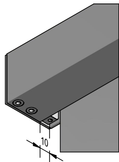
Detail A Stoffauslass
