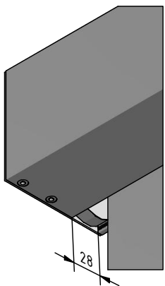
Detail A Stoffauslass
