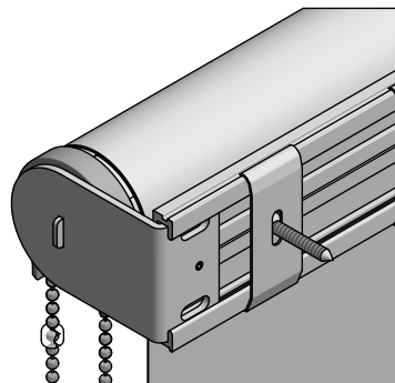
Montage: Montageleiste mit Montageclip
