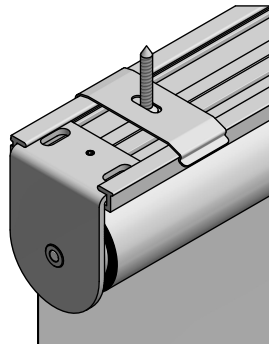
Montage: Montageleiste mit Montageclip
