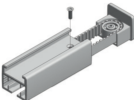
Umlenkung Glydea „Mini“
