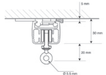
Montage mit Deckenclip
