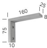
Wandträger 16 cm
