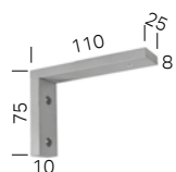
Wandträger 11 cm
