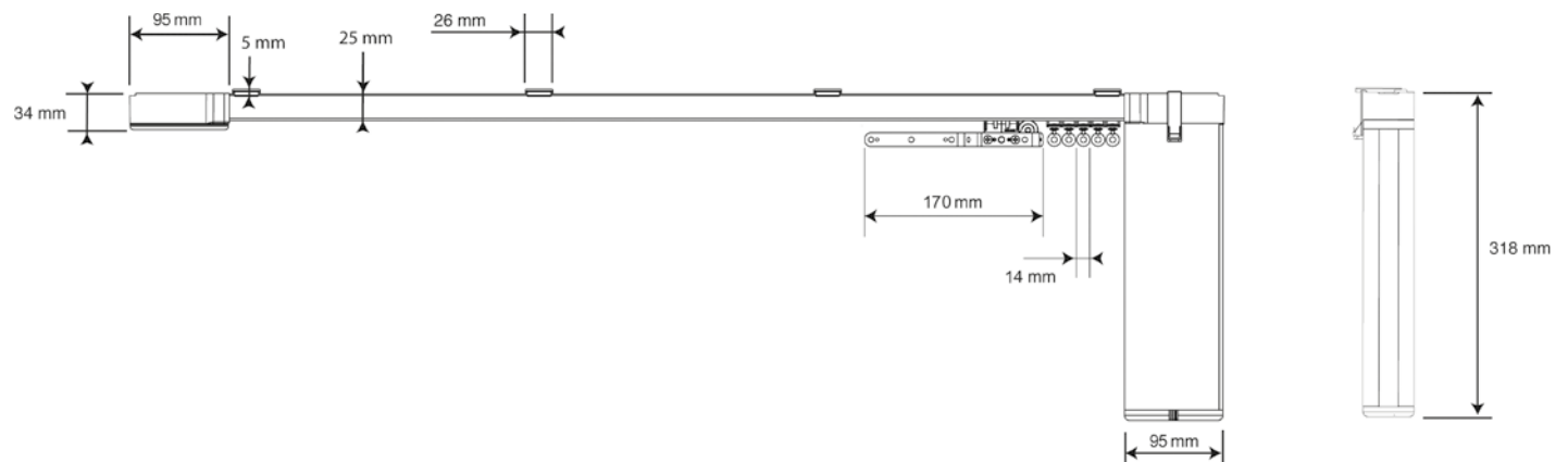
Seitenansicht
