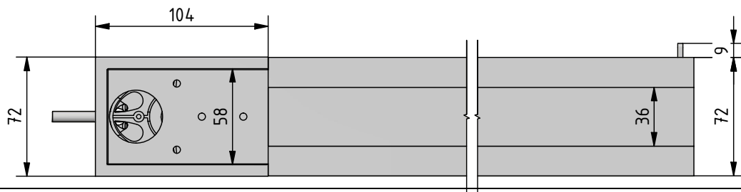
Durach Sonnenschutz | Blendschutz | Raumakustik Durach GmbH Alte Bahnlinie 20 D-88299 Leutkirch Telefon: +49(0)7567 988 84-0 Telefax: +49(0)7567 988 84-20 e-mail: Info@durach.com Internet: www.durach.com Maßstab 1 : 3,25 Material: Alu, V2A DATUM Name Benennung: Glydea-595-Mini-in-Einbauprofil-Ansichtszeichnung Glydea-595-Elektrozugschiene mit "Mini"-Umlenkung Montage in Einbauprofil P-8050 Gezeichnet 01.02.2023 Robert Lobinger Geändert 29.07.2025 Robert Lobinger Norm Hinweis: Zeichnungsnummer: 2023.007.001.003 Deckenmontage 1 A4 Status Änderungen DATUM Name Diese Zeichnung ist geistiges Eigentum der Fa. Durach GmbH und darf ohne unser Einverständnis weder kopiert noch Dritten Personen mitgeteilt noch anderweitig benutzt werden.
