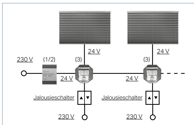
(1) Power 2,7 DC Trafo Gruppennetzteil bis zu 6 Antriebe
