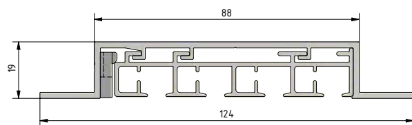
4-läufig
