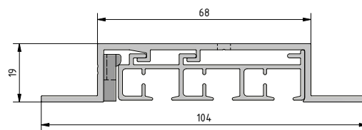
3-läufig
