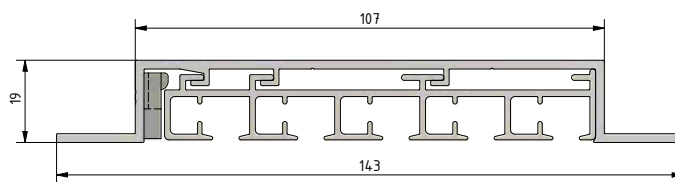
5-läufig
