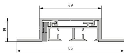
2-läufig
