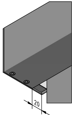
Detail A Stoffauslass
