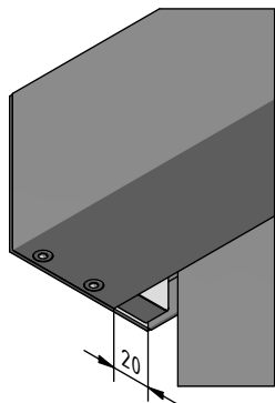
Detail A Stoffauslass
