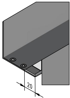
Detail A Stoffauslass
