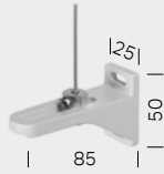
Seilverspannung für Wandmontage lang
