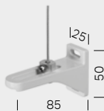
Seilverspannung für Wandmontage
