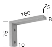
Wandträger 16 cm
