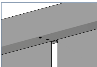
E-200-Z Zwischenträger
