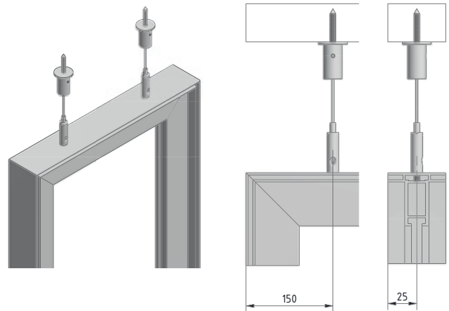
Seilabhängung
