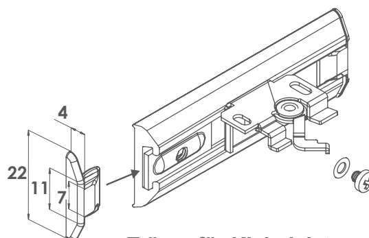
Träger für Klebeleiste mit Halteplatte oben
