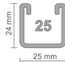
Oberschiene 25
