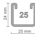
Oberschiene 25
