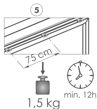
Träger für Klebeleiste Verspannung unten
