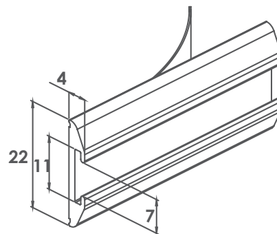
Klebeleiste aus Aluminium Farben: Weiß, silber
