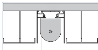
Einbau in abgehängte Decke aus Metall (MP-80-V2)
