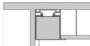
Einbau in abgehängte Decke Wand-/ Fassadenbündig (MP-80-V3)
