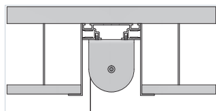
Einbau in abgehängte Decke (MP-80-V1)
